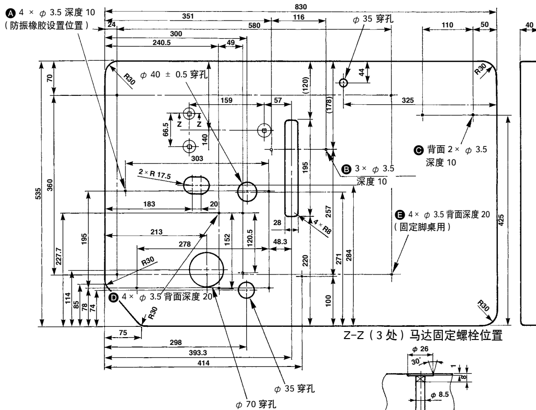
机台参考图
