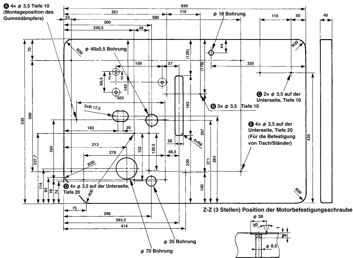
Tischplatten-Maßzeichnung als Referenz
