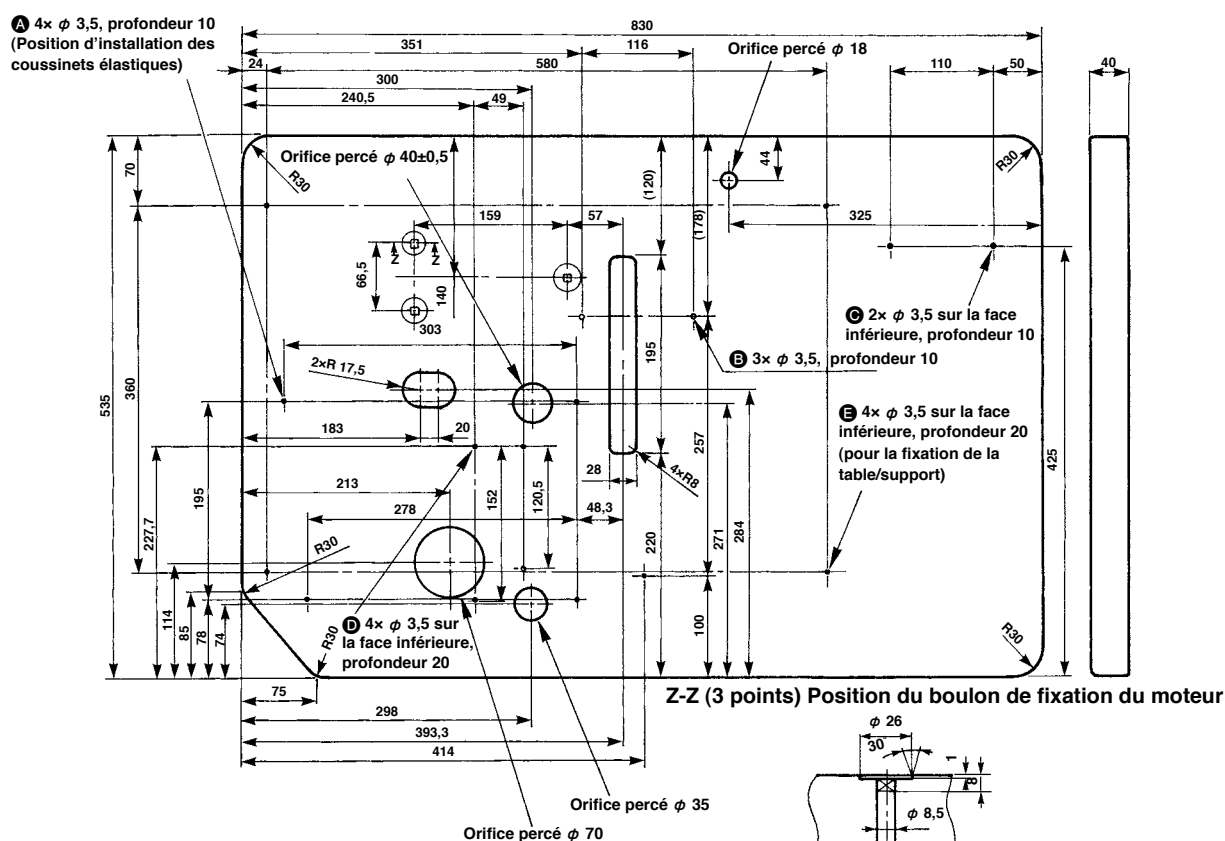
Plan de référence de la table
