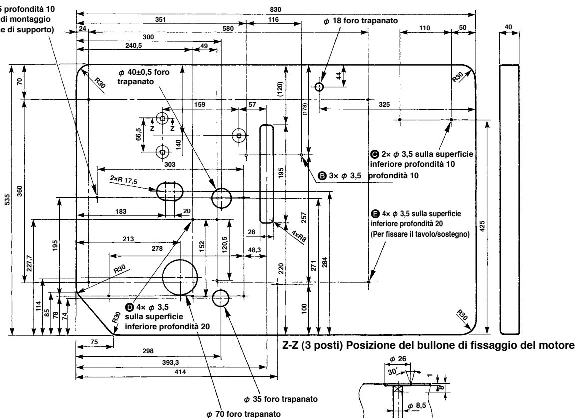
Disegno di riferimento del tavolo
